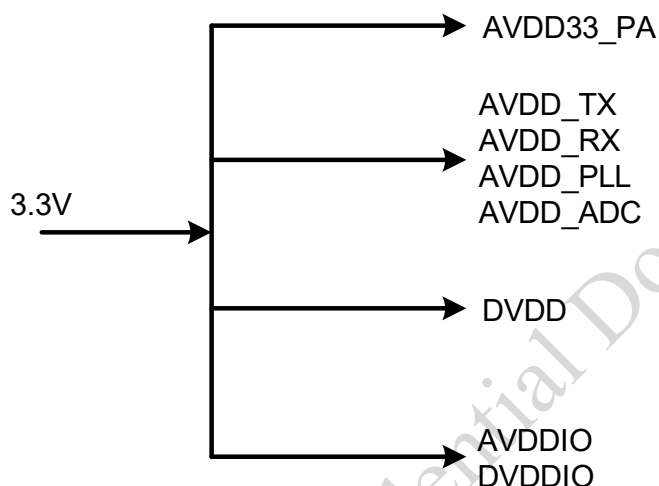
图 3 3.3V 单供电
