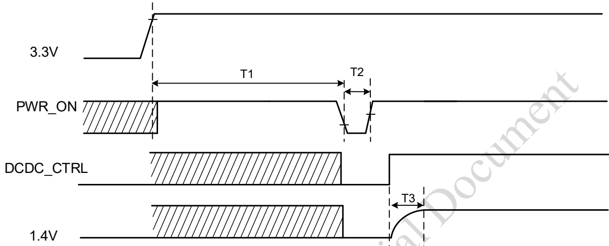
图 5 GPIO 控制 PWR_ON 的上电时序图
