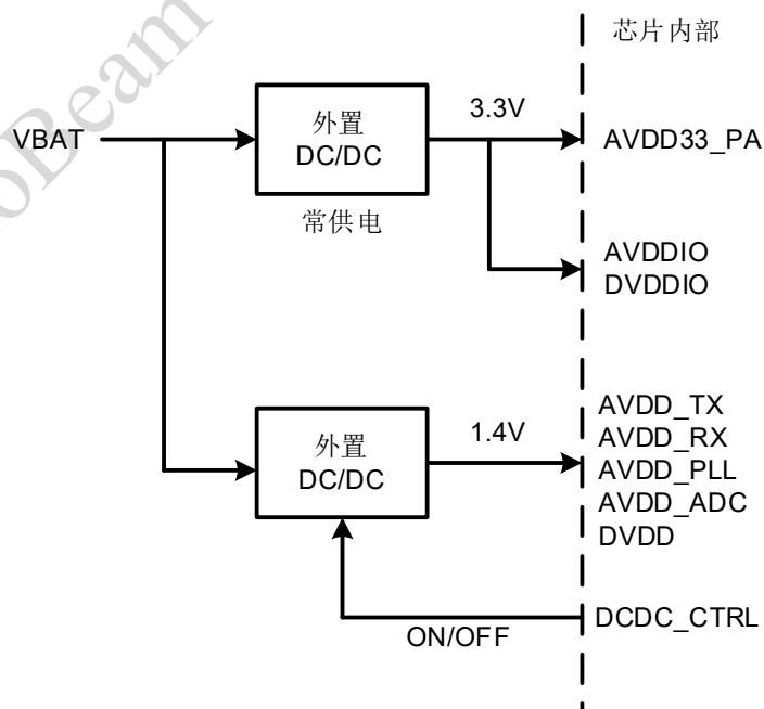
图 4 低功耗电池供电
