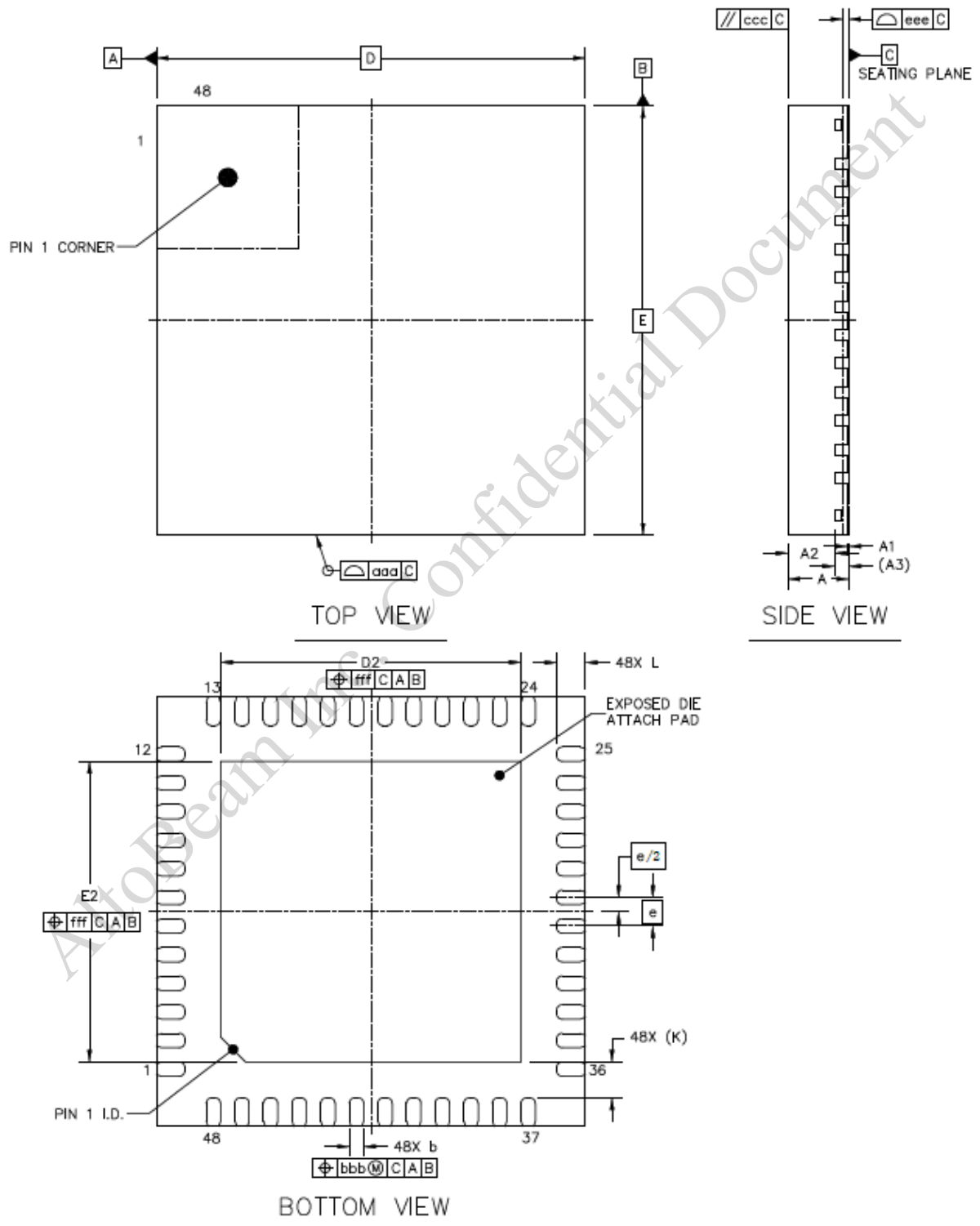
图 8 ATBM6441 封装图
