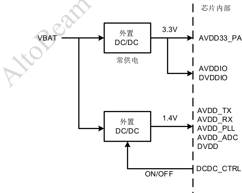
图 4 低功耗电池供电
