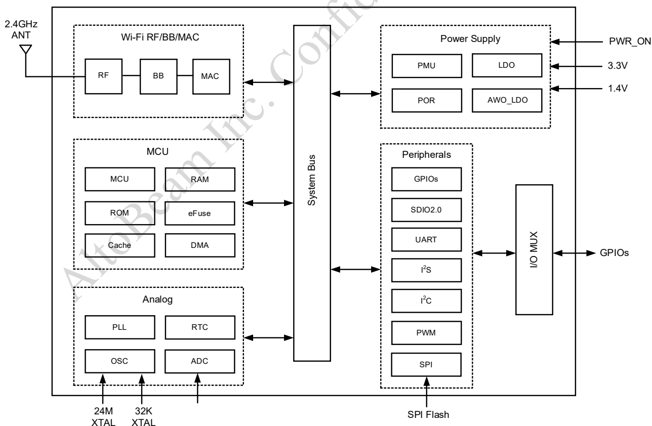
图 1 ATBM6441 框图
