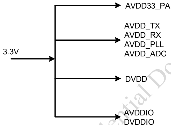
图 3 3.3V 单供电
