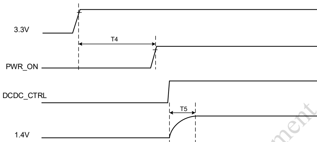
图 6 RC 电路控制 PWR_ON 的上电时序图
