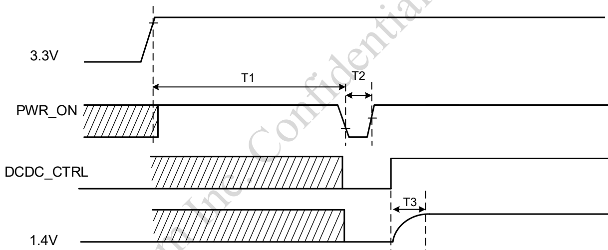
图 5 GPIO 控制 PWR_ON 的上电时序图
