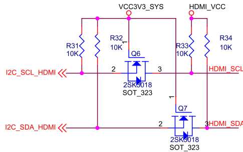
I2C Level Shift
