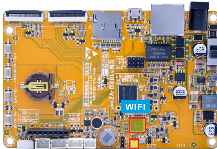
WiFi_ANT
